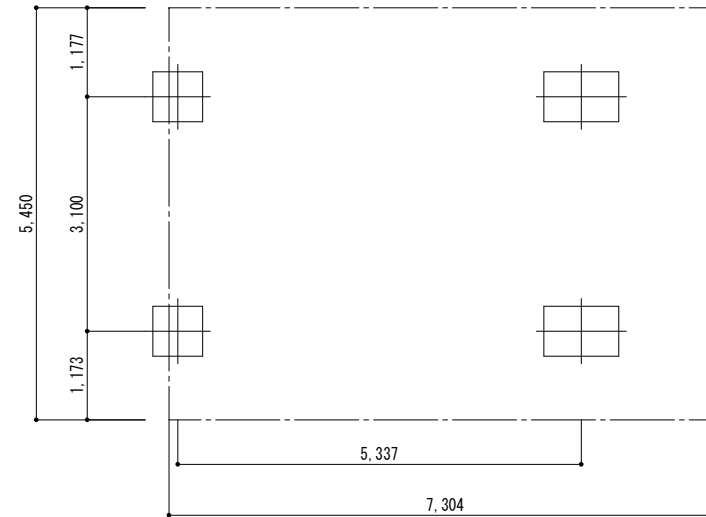
■ 基礎配置図
